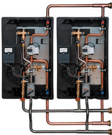
tubra®-FRISTA KL + Verrohrungsset
