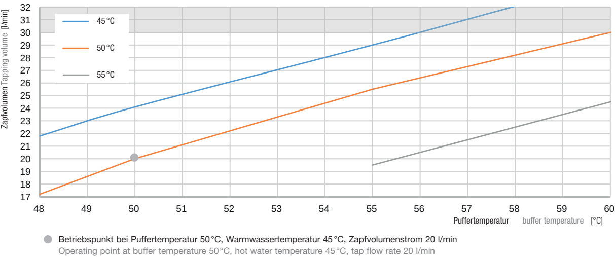
Elektronische Trinkwasserstation tubra ® -FS-C M Zapfvolumen bis 41 l/min, Puffertemperatur von 50 °C bis 60 °C Electronic drinking water station tubra ® -FS-C M tapping volume up to 41 l/min, buffer temperature of 50 °C to 60 °C
