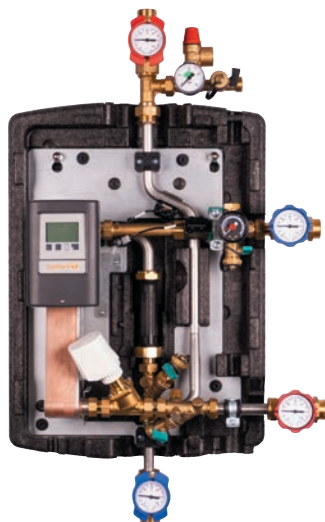
tubra® - DHG, ohne Pumpe
